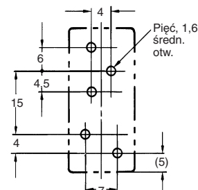
Otworki montażowe
