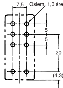
Otworki montażowe
